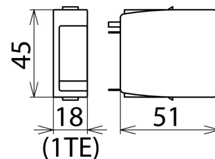
Rozměry DR MOD 255
