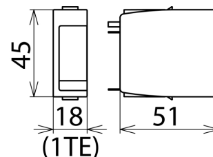
Rozměry DR MOD 150
