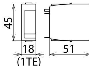
Rozměry DR MOD 75
