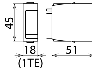
Rozměry DR MOD 60
