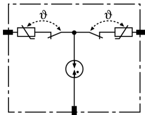
Schéma vnitřního zapojení DR MOD 60
