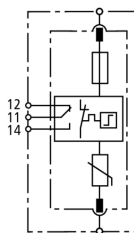
Schéma vnitřního zapojení DG SE CI WE 440 FM
