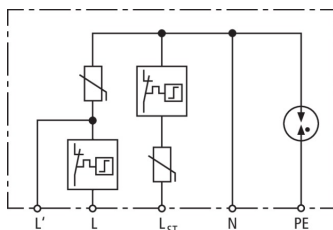
Schéma vnitřního zapojení DCOR L 3P 275 SO IP
