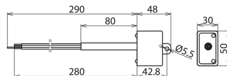
Rozměry DCOR L 3P 275 SO IP
