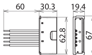
Rozměry DCOR L 3P 275 SO LTG
