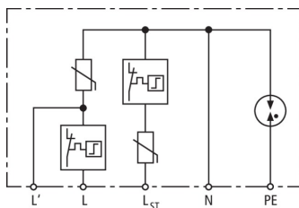
Schéma vnitřního zapojení DCOR L 3P 275 SO LTG
