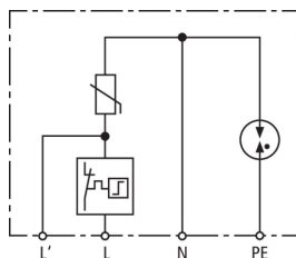
Schéma vnitřního zapojení DCOR L 2P 275 SO LTG
