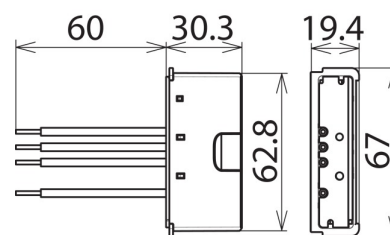
Rozměry DCOR L 2P 275 SO LTG
