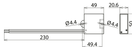
Rozměry DCOR L 1P 275
