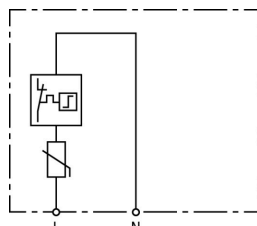
Schéma vnitřního zapojení DCOR L 1P 275
