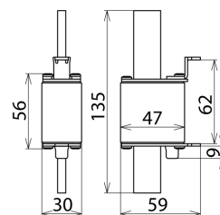
Rozměry VA NH1 280
