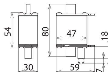
Rozměry V NH00 280 FM
