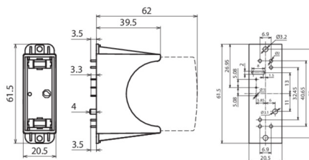
Rozměry DG PCB I 275 FM
