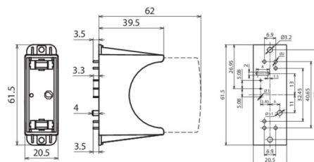
Rozměry DG PCB PV I 500 FM
