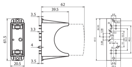
Rozměry DG PCB 385 FM
