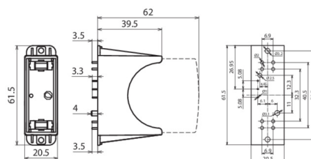
Rozměry DG PCB PV 300 FM
