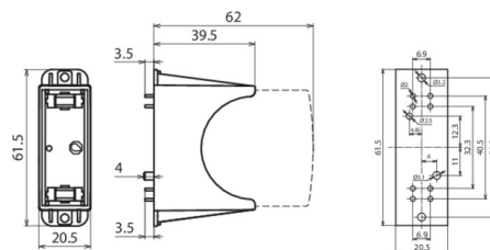
Rozměry DG PCB PV 300
