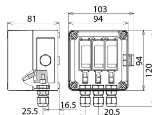
Rozměry DCU YPV SCI 1000 1M
