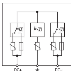
Schéma vnitřního zapojení DCU YPV SCI 1000 1M
