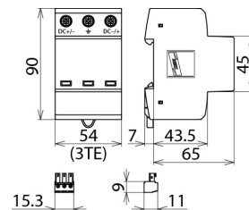
Rozměry DG YPV SCI 600 FM
