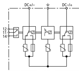
Schéma vnitřního zapojení DG YPV SCI 600 FM
