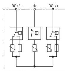
Schéma vnitřního zapojení DG YPV SCI 1000
