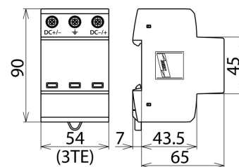
Rozměry DG YPV SCI 1000
