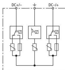
Schéma vnitřního zapojení DG YPV SCI 600
