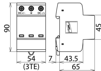
Rozměry DG YPV SCI 600
