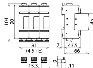
Rozměry DG ME YPV SCI1500 FM
