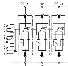
Schéma vnitřního zapojení DG ME YPV SCI1500 FM
