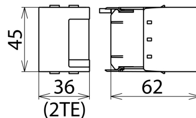
Rozměry DSE MOD 60
