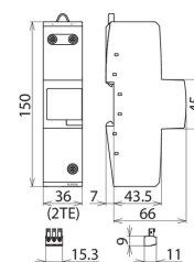
Rozměry DBM 1 760 FM
