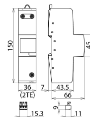
Rozměry DBM 1 440 FM
