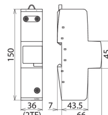
Rozměry DBM 1 440
