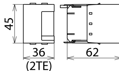
Rozměry DB M MOD 150
