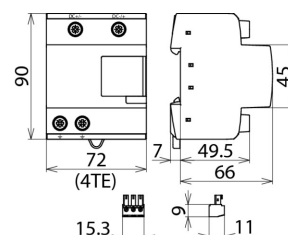
Rozměry DCB YPV 1500 FM
