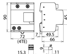
Rozměry DCB YPV 1200 FM
