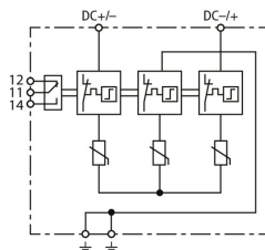
Schéma vnitřního zapojení DCB YPV 1200 FM
