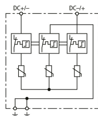
Schéma vnitřního zapojení DCB YPV 1500
