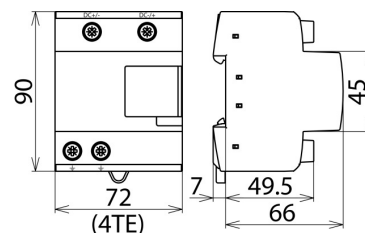
Rozměry DCB YPV 1500
