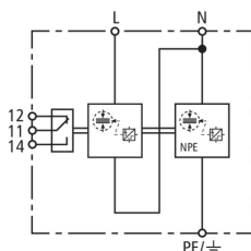
Schéma vnitřního zapojení DSH B TT 2P 255 FM
