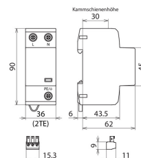
Rozměry DSH B TT 2P 255 FM
