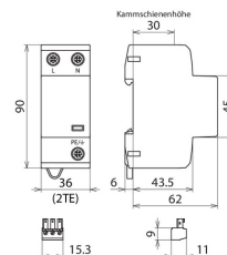
Rozměry DSH TT 2P 255 FM
