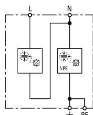
Schéma vnitřního zapojení DSH TT 2P 255
