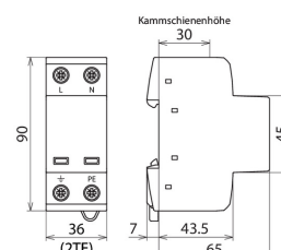
Rozměry DSH TT 2P 255
