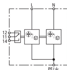
Schéma vnitřního zapojení DSH B TN 255 FM
