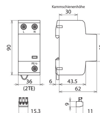
Rozměry DSH B TN 255 FM
