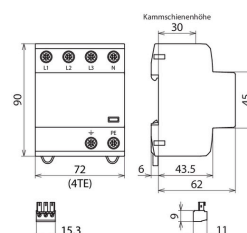
Rozměry DSH B TT 255 FM
