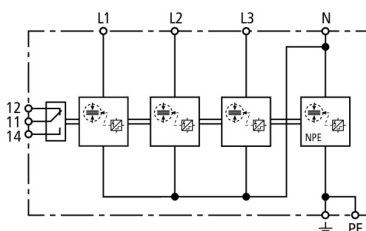
Schéma vnitřního zapojení DSH B TT 255 FM
