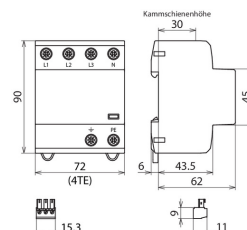
Rozměry DSH TT 255 FM
