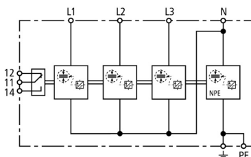
Schéma vnitřního zapojení DSH TT 255 FM
