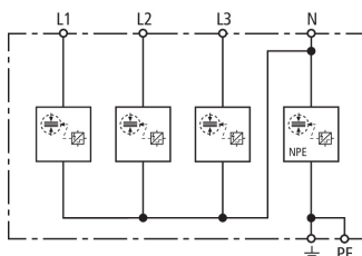
Schéma vnitřního zapojení DSH TT 255
