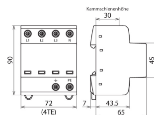
Rozměry DSH TT 255
