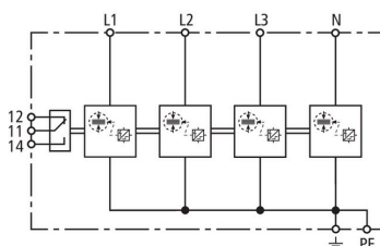
Schéma vnitřního zapojení DSH TNS 255 FM
