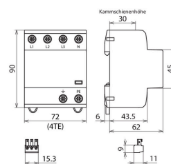
Rozměry DSH TNS 255 FM
