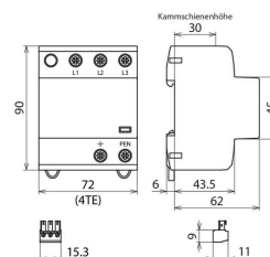
Rozměry DSH B TNC 255 FM
