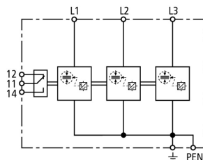
Schéma vnitřního zapojení DSH B TNC 255 FM
