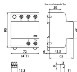
Rozměry DSH TNC 255 FM
